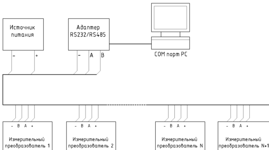
Рис.4. Схема подключения измерительных преобразователей.
