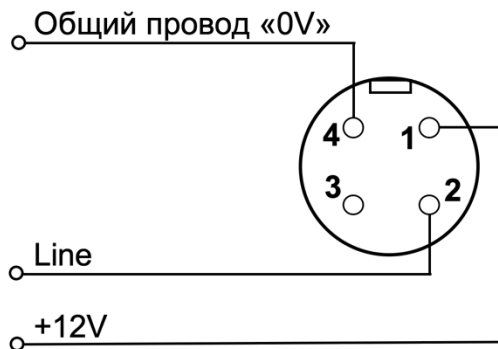
Рис.5. Схема «распайки» кабеля (вид со стороны «распайки» розетки) для подключения ДВ2ТСМ-6Т-1П-Г.
