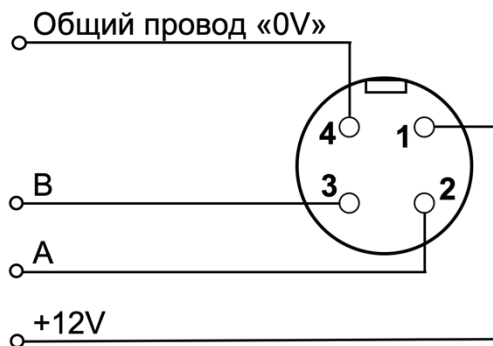
Рис.3. Схема «распайки» кабеля (вид со стороны «распайки» розетки) для подключения ДВ2ТС-6Т-1П-Г.
