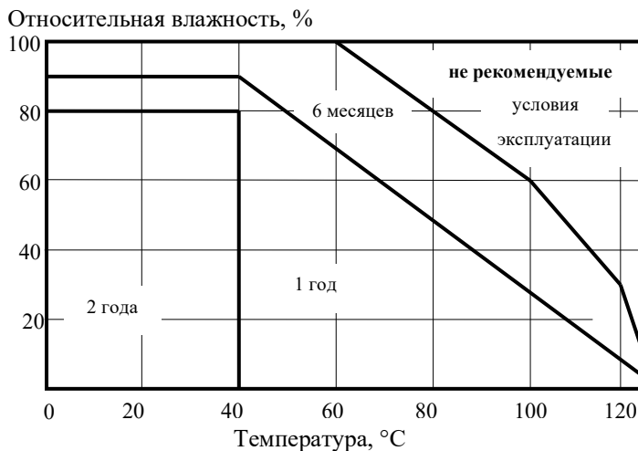
Рис.2. Зависимость рекомендуемой периодичности юстировки от условий эксплуатации преобразователя.
