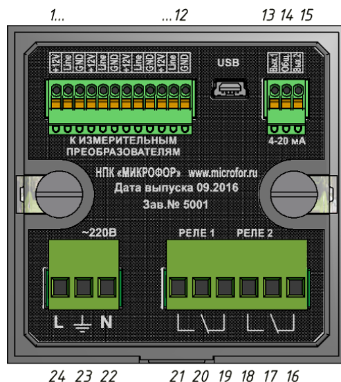
Рис.9. Вид задней панели блока индикации.
