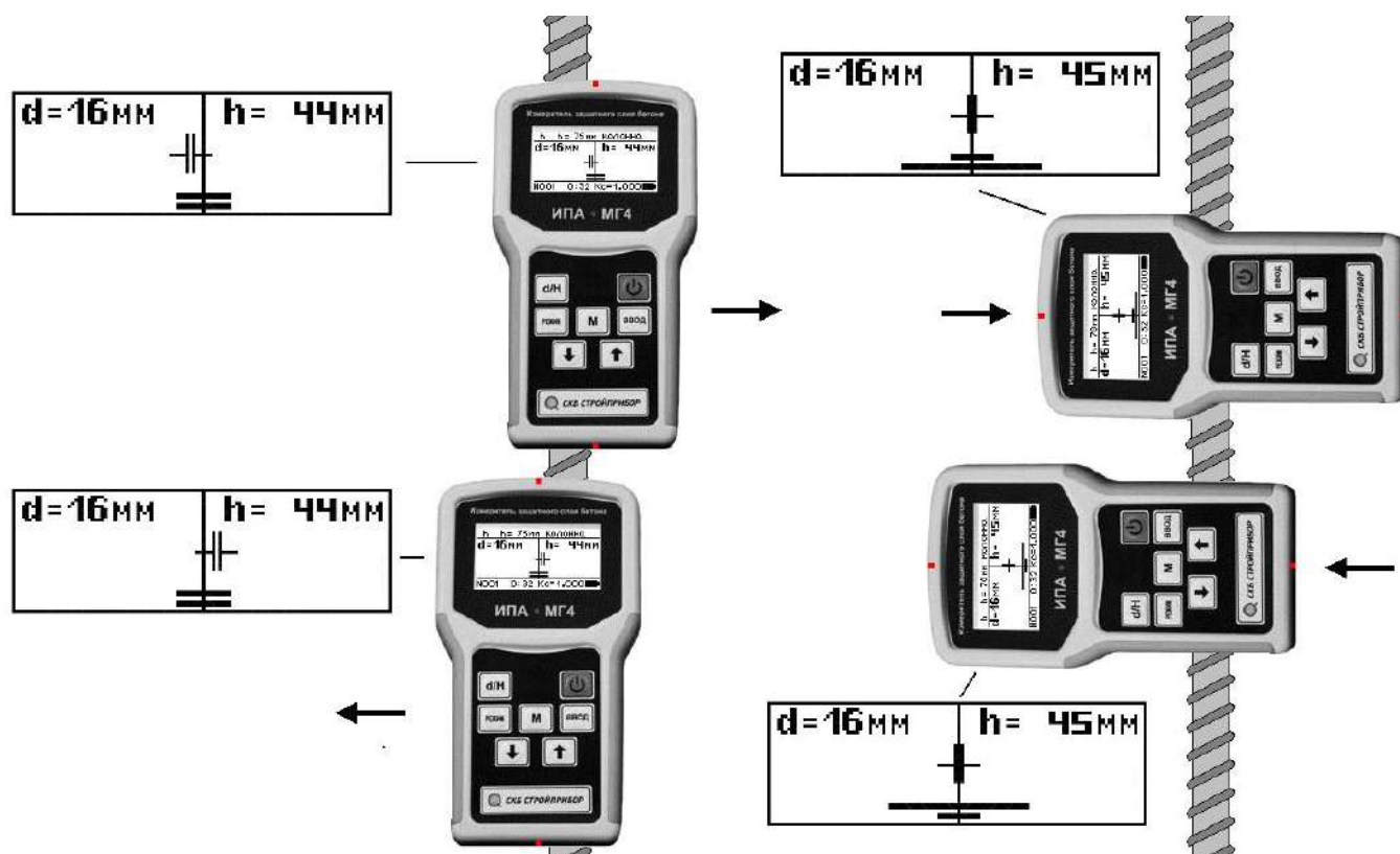
Рисунок 3 – Определение оси арматурного стержня при повороте измерителя на 90^\circ
