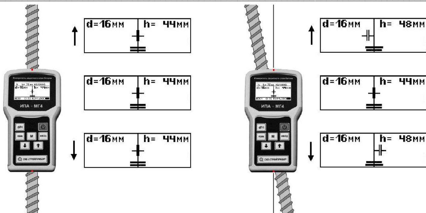
Рисунок 2 – Определение оси арматурного стержня.
