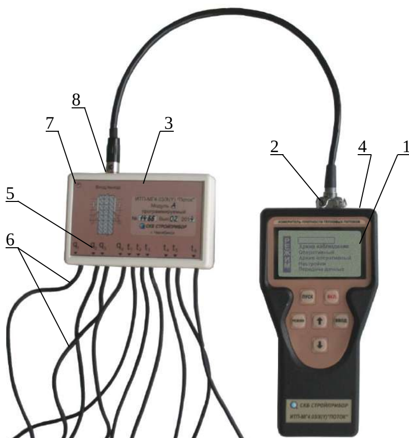
Рисунок 1.1 – Общий вид измерителя ИТП-МГ4.03/10(І) «ПОТОК»
