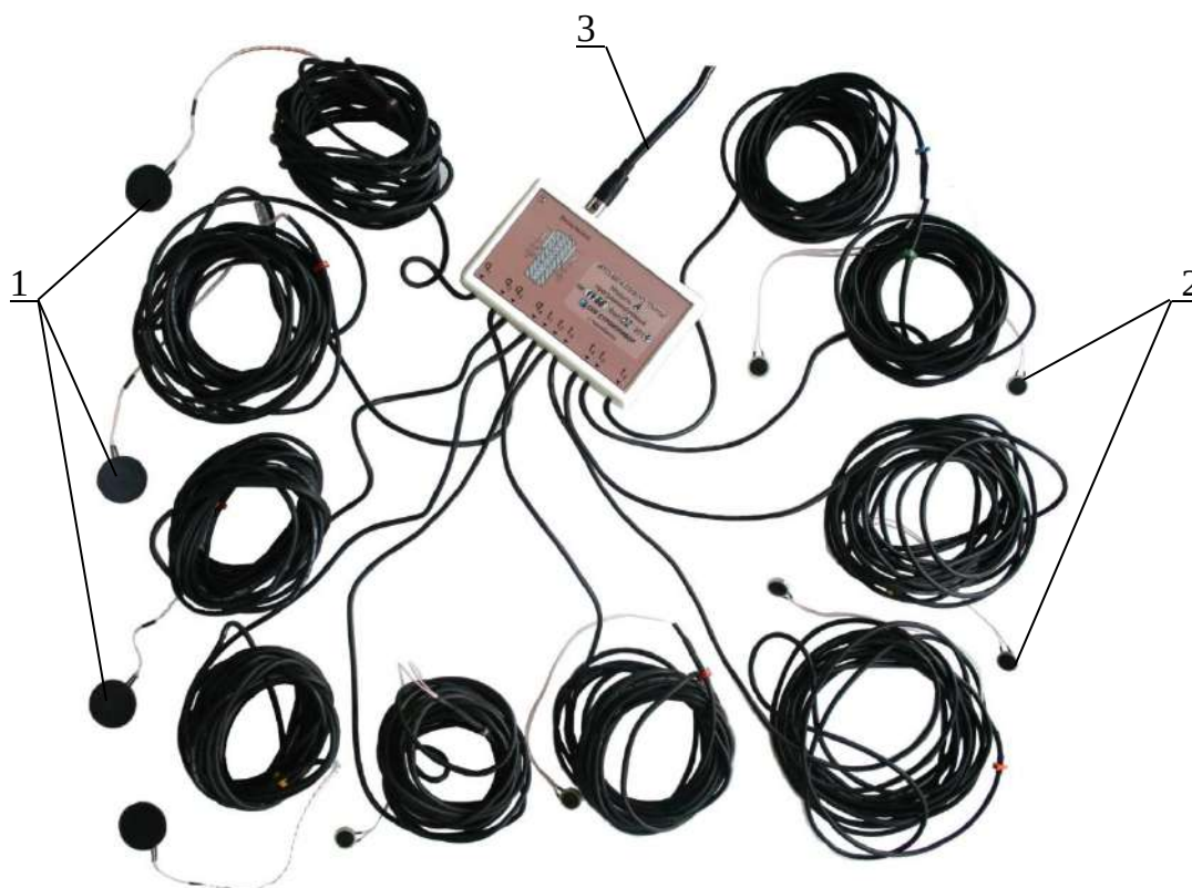
1 – датчики теплового потока; 2 – датчики температуры; 3 – кабель связи с электронным блоком
