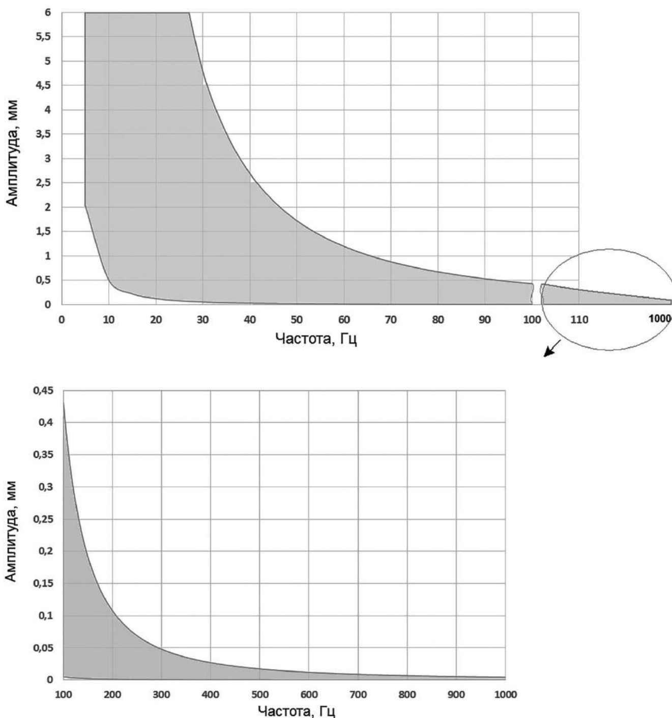
Рисунок 1.2 – Зависимость диапазона измерения амплитуды виброперемещения от частоты колебаний объекта контроля
