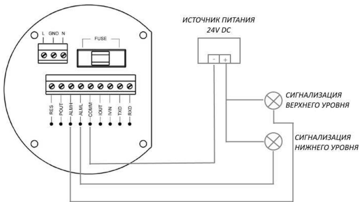
Рисунок 10. Аварийная сигнализация ВП MT200HC / MT206
