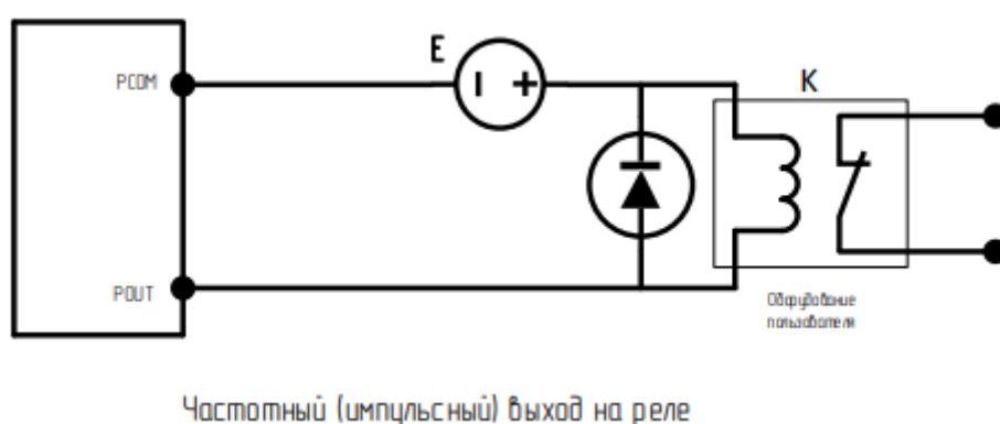
Рисунок 9 – Выход для реле
