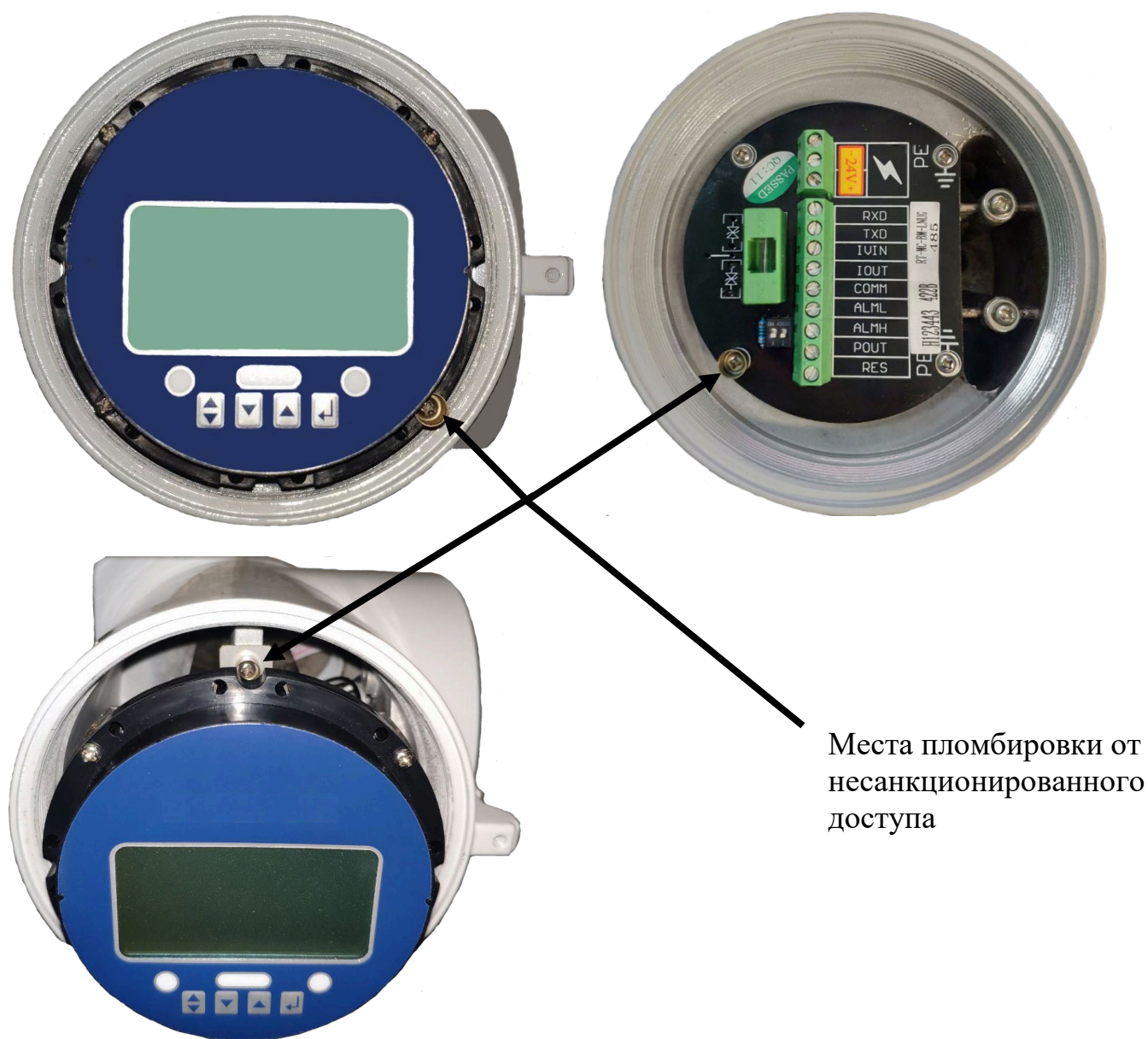
Рисунок 13. Схема пломбировки ВП MT200HC / MT206
