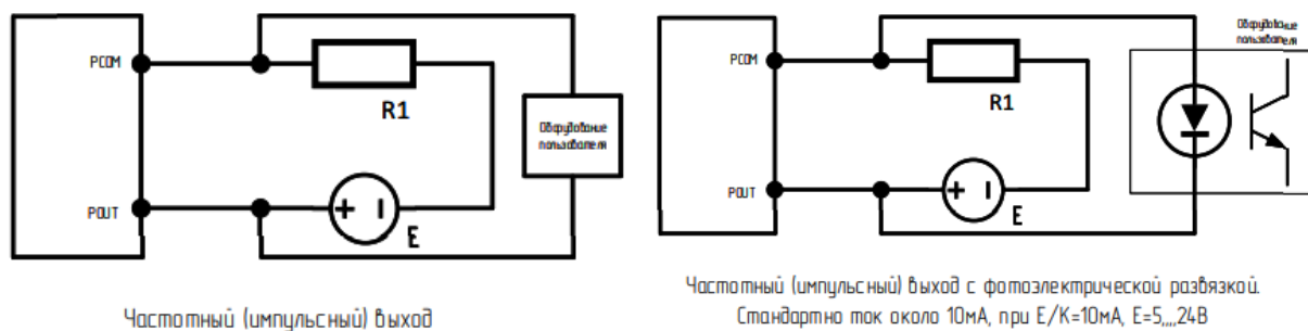
Рисунок 8 – Частотный (импульсный) выход
