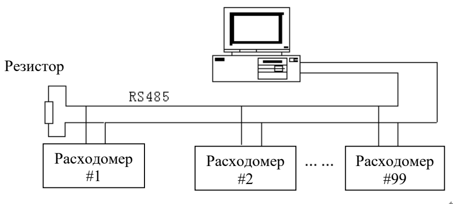
Рисунок 15. Структура сети расходомера
