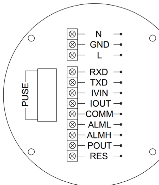
Рисунок 3. Электрическая схема ВП MT200HC / MT206
