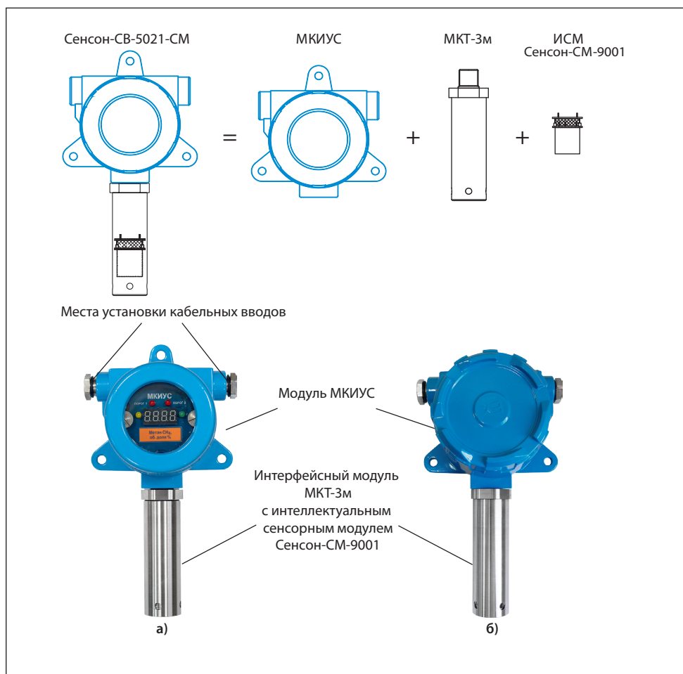
Рис.1. "Сенсон-СВ-5021" в базовом исполнении (а) и исполнение без индикатора (б)
