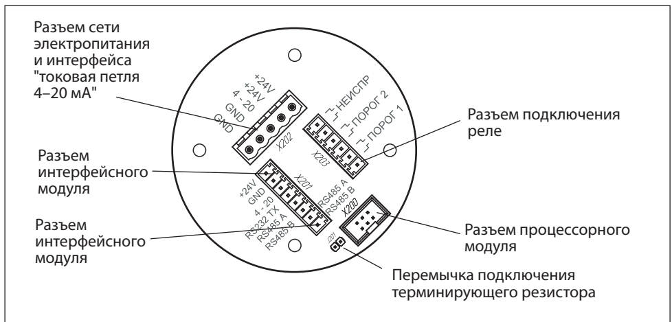
Рис.12. Модуль коммутации
