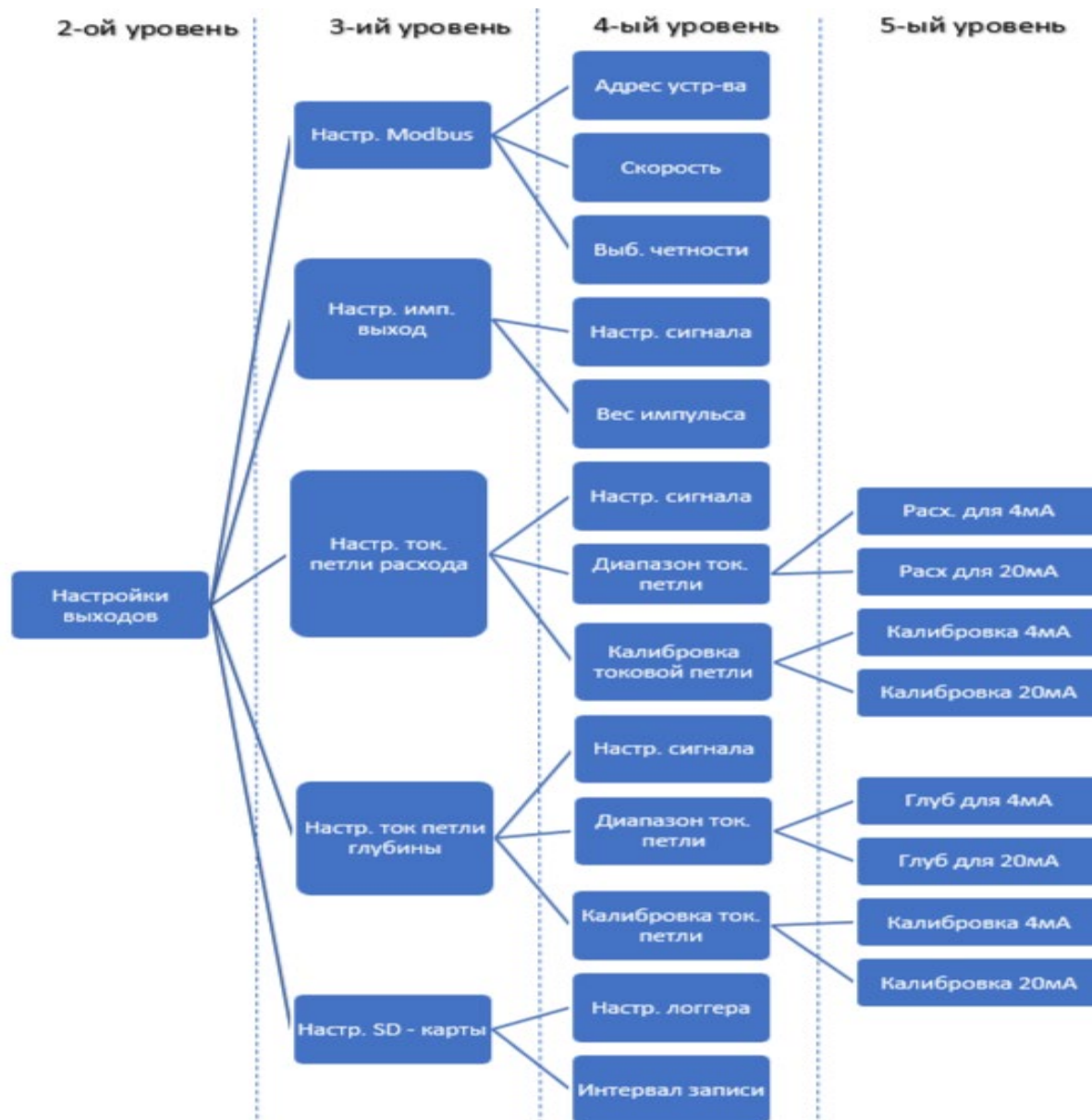
Рисунок 5.12. Структура пункт меню «Настройки выходов»
