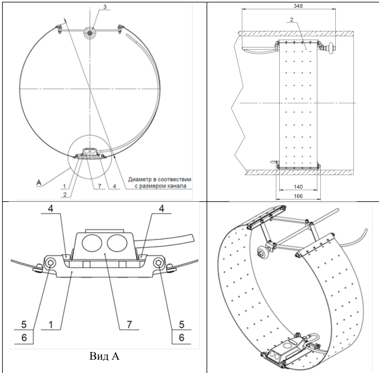
Рисунок 4.6. Монтажный комплект и расположение зонда на монтажной площадке.
