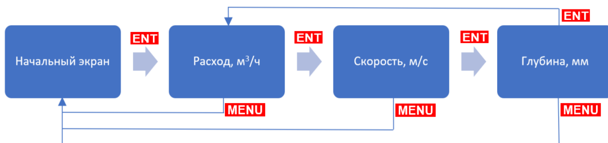
Рисунок 5.2. Вывод на экран отдельных значений характеристик потока жидкости
