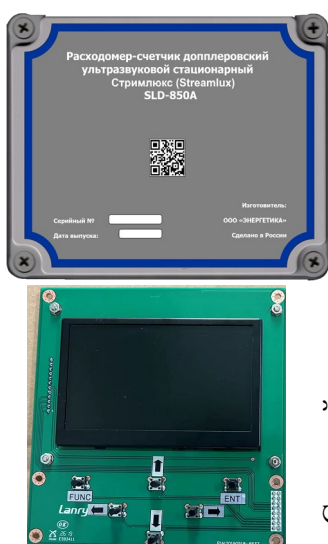
SLD-850A – автономный со съемным экраном
