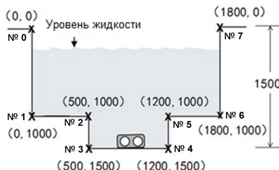
Рисунок 5.9. Поперечное сечение канала с заданными координатами контрольных точек
