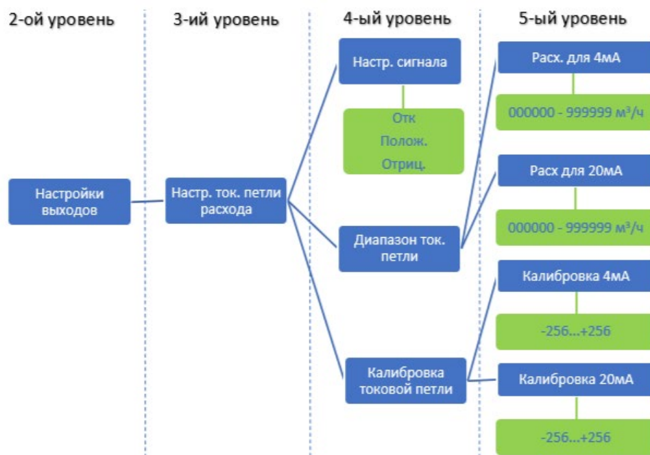
Рисунок. 5.15. Настройка токовой петли расхода
