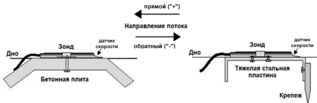
Рисунок 4.4. Монтаж зонда расходомера в открытом канале / русле
