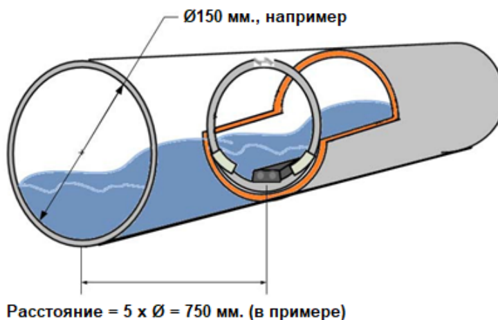
Рисунок 4.5. Расположение зонда в трубе
