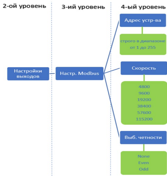
Рисунок. 5.13. Настройка протокола Modbus
