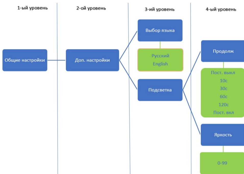
Рисунок. 5.19. Установка языка и яркости
