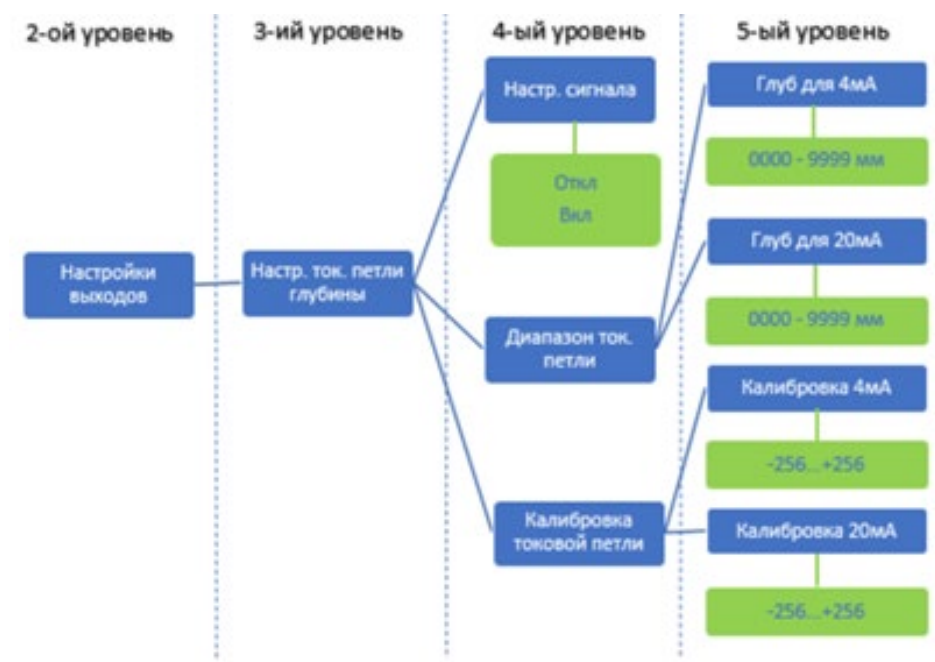
Рисунок. 5.16. Настройка токовой петли глубины
