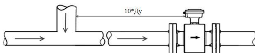
Рисунок 12. Расстояние от точки смешивания потоков
