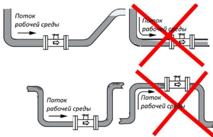
Рисунок 10. Монтаж на горизонтальном трубопроводе
