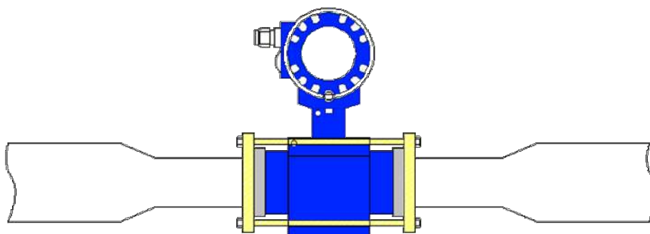
Рисунок 15.2. Соединение сэндвич
