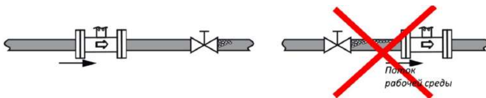
Рисунок 11. Монтаж расходомера с трубопроводной арматурой
