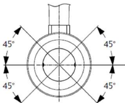
Рисунок 14. Расположение электродов
