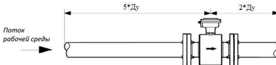
Рисунок 7. Прямые участки
