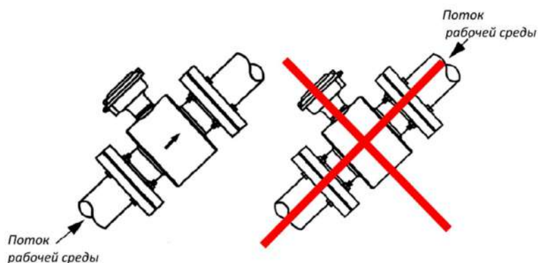
Рисунок 9. Монтаж на наклонном трубопроводе
