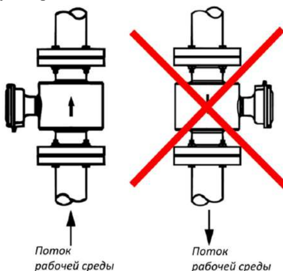
Рисунок 8. Монтаж на вертикальном трубопроводе
