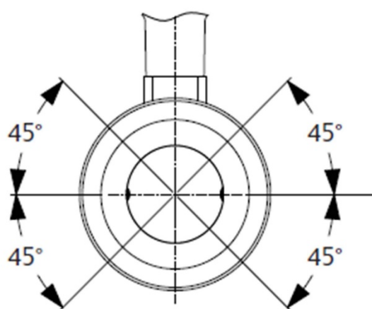
Рисунок 14. Расположение электродов
