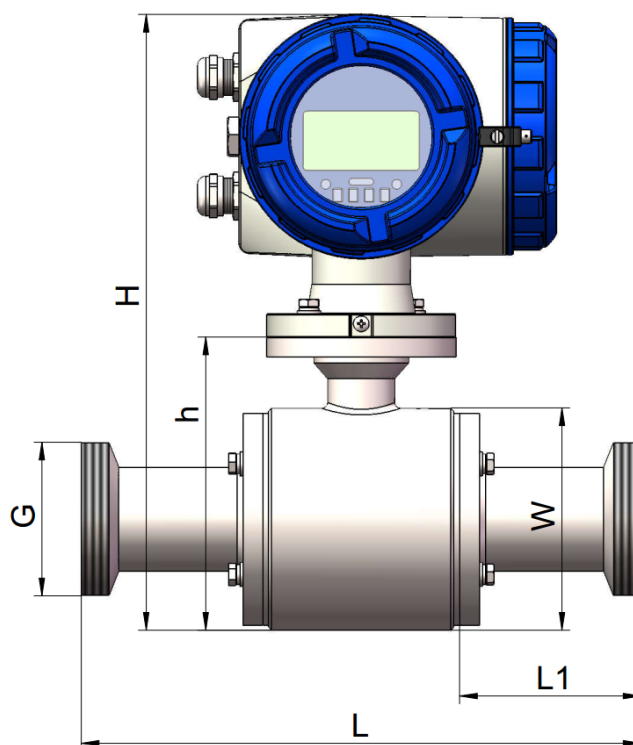
Рисунок 2.2. Габаритные размеры первичного преобразователя (тип соединения – молочная гайка)
