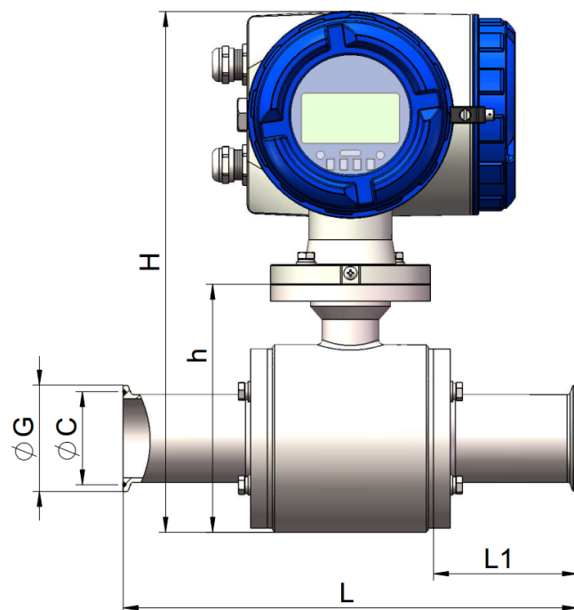
Рисунок 2.1. Габаритные размеры первичного преобразователя (тип соединения – кламп)
