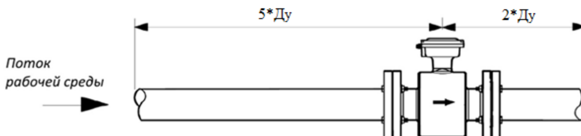
Рисунок 7. Прямые участки
